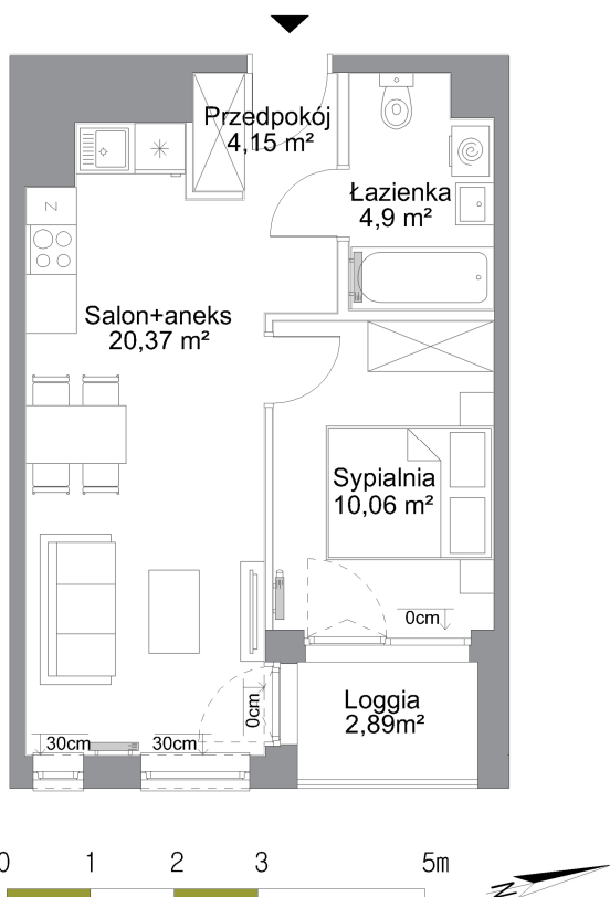
RZUT KONDYGNACJI
