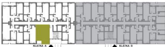
RZUT KONDYGNACJI
